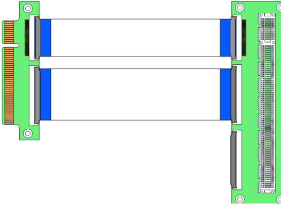
P25S-P27F (KZ-B23x8-DB23)
